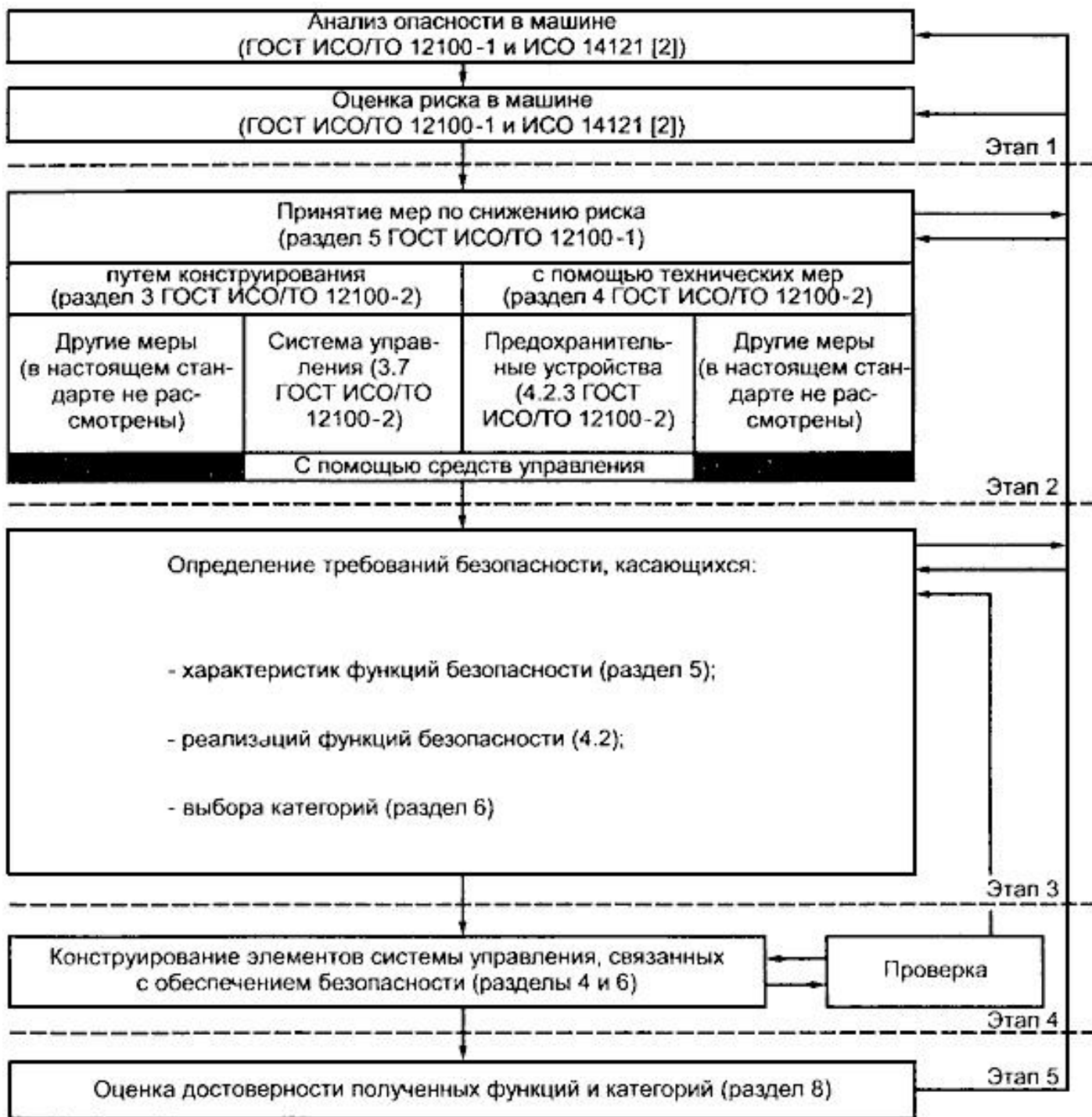
Рисунок 1 - Итеративный процесс при конструировании элементов системы управления, связанных с обеспечением безопасности
